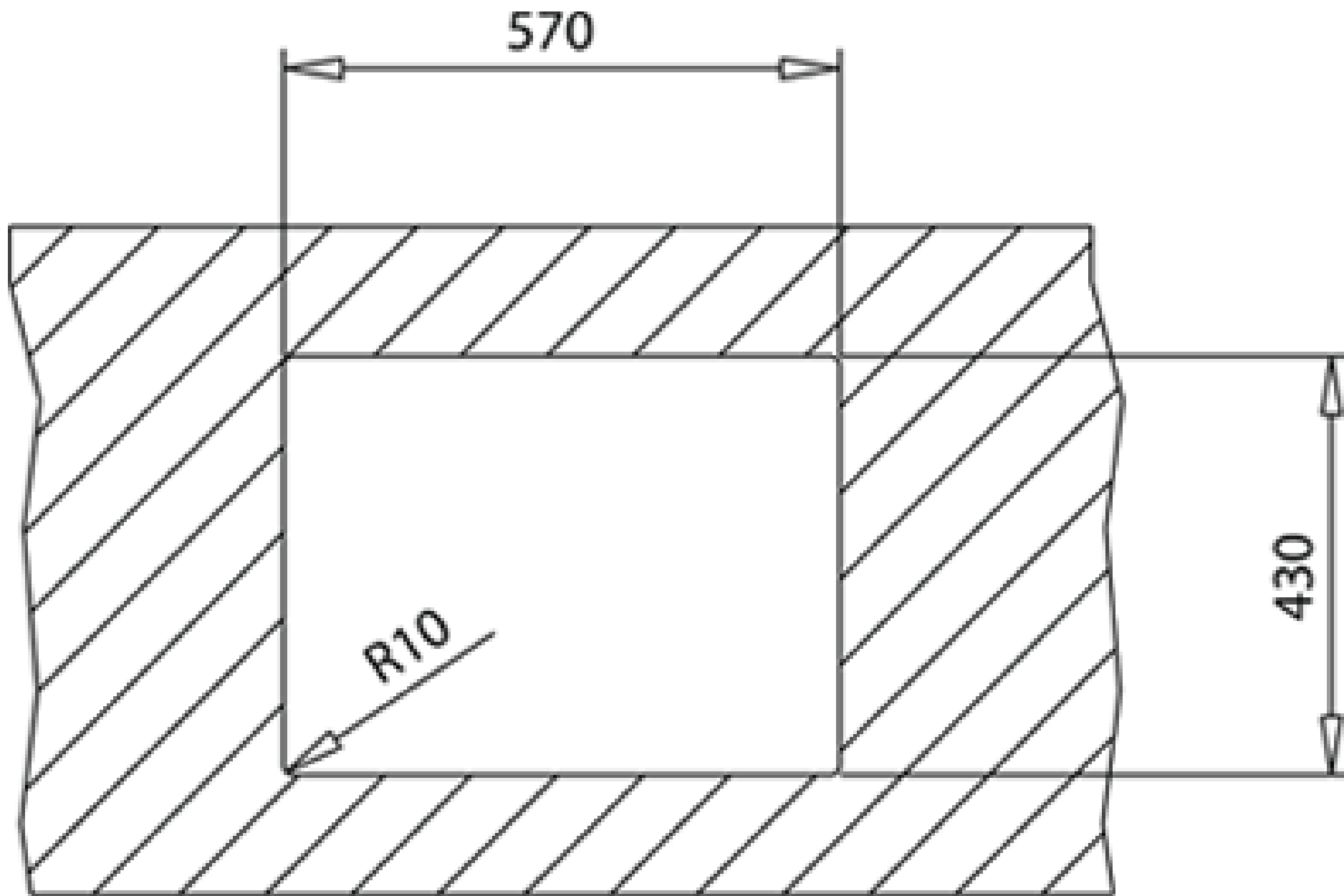
Ausschnitt für aufliegende Spüle
