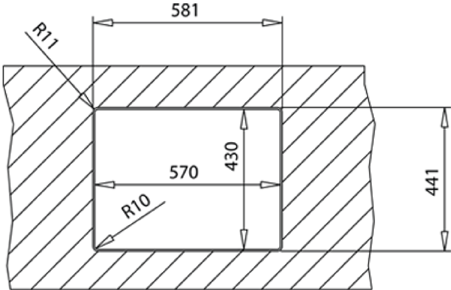
Ausschnitt für flächenbündige Spüle
